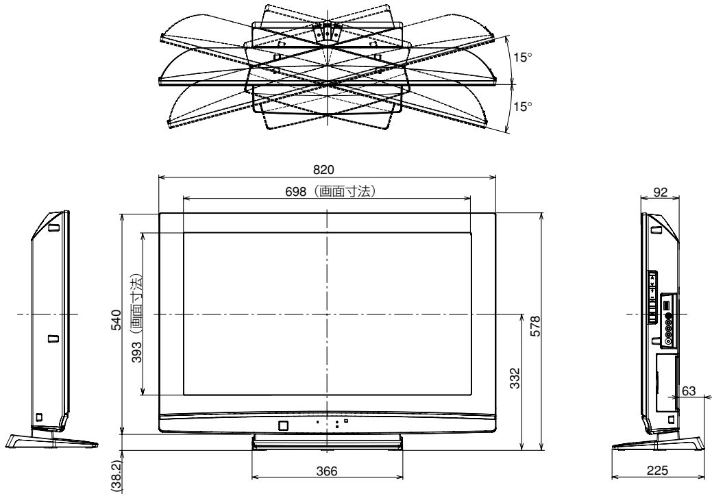
据え置き設置用スタンド取付時
