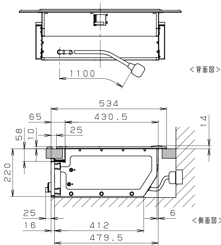
<キッチン加工寸法図>
