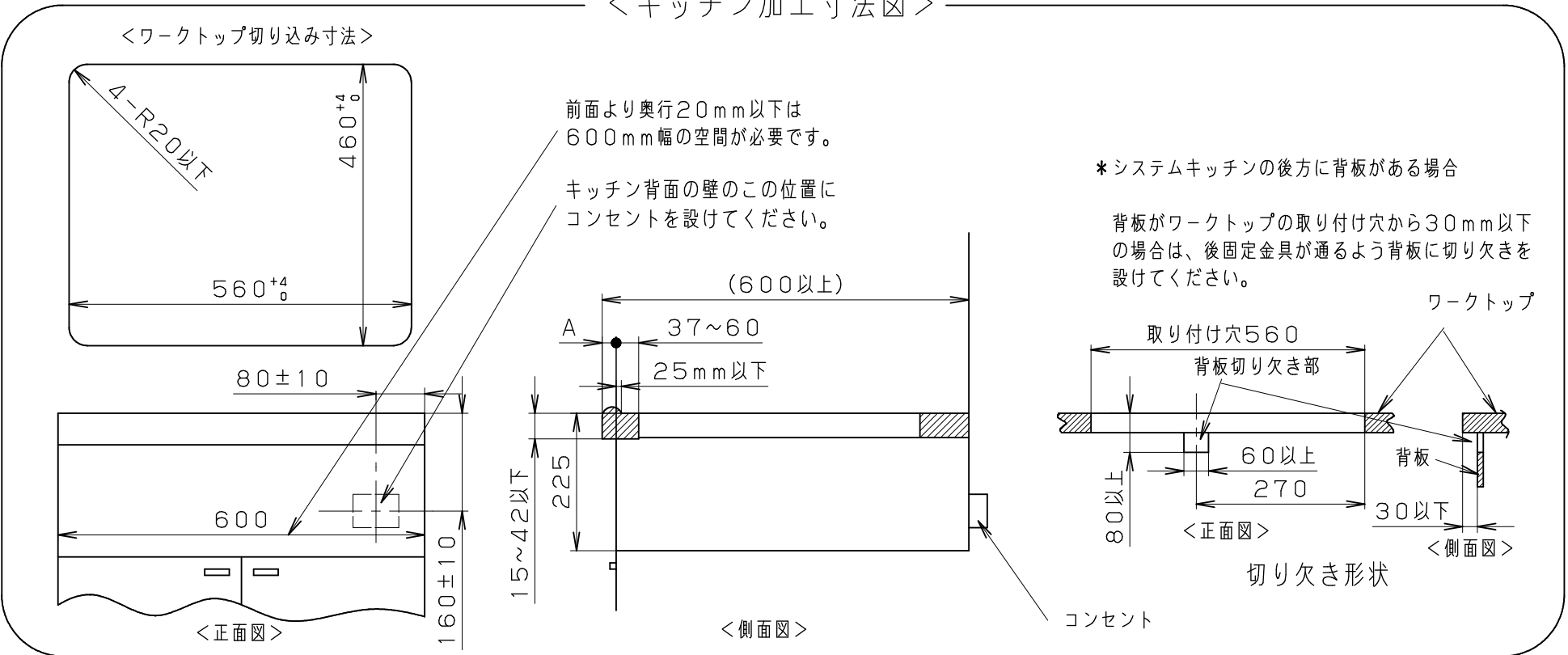
<キッチン加工寸法図>
