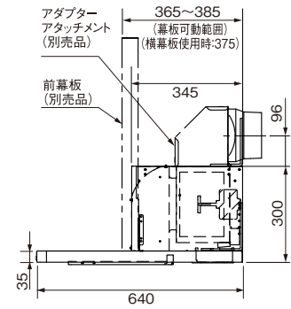
(右側面図)
