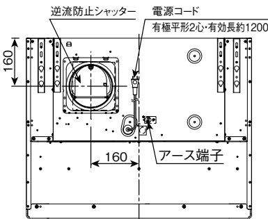
(平面図)
