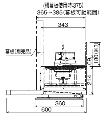
(右側面図)
