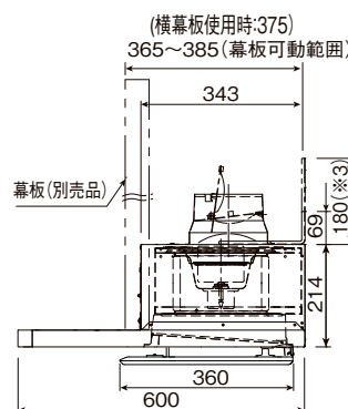
(右側面図)
