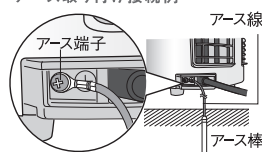
アース取り付け接続例
