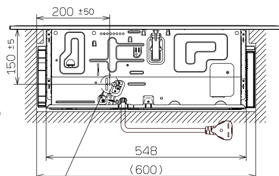
背面図
