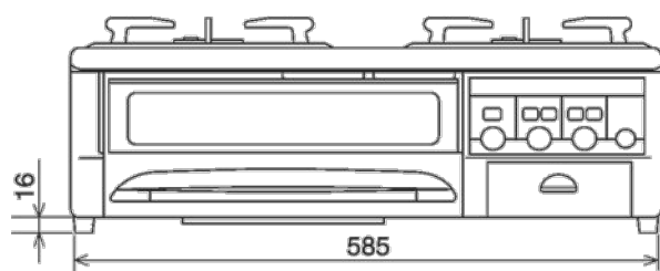
正面図
