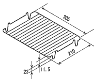
焼網 (グリル網)
