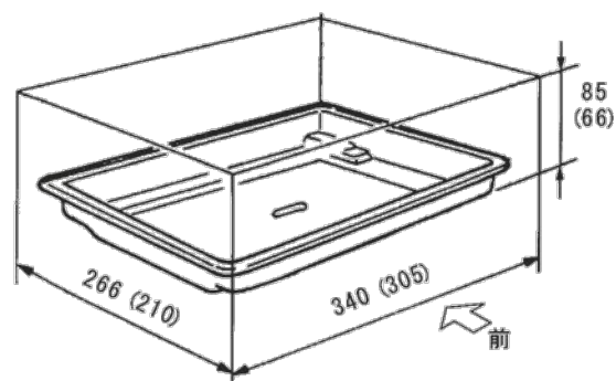
グリル庫内寸法
