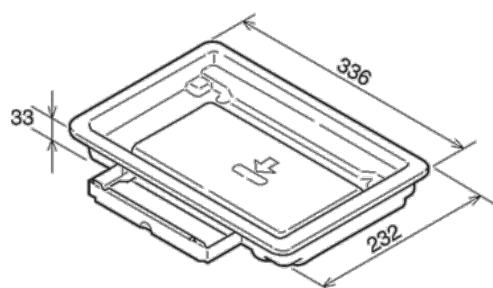
グリル水入れ皿
