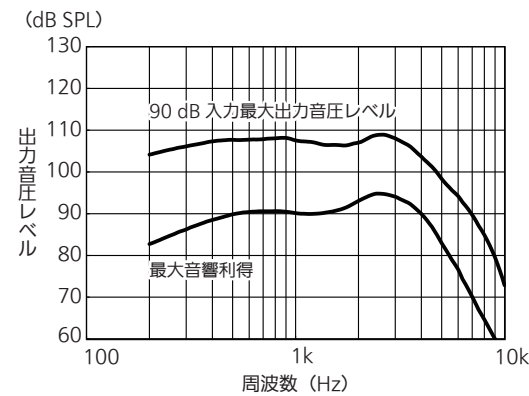
90 dB 入力最大出力音圧レベル周波数レスポンスと 最大音響利得周波数レスポンス
