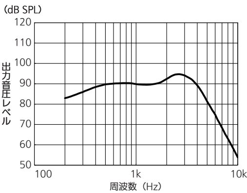
規準周波数レスポンス
