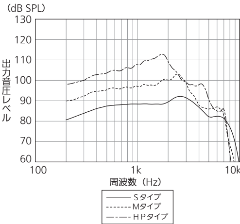
規準周波数レスポンス
