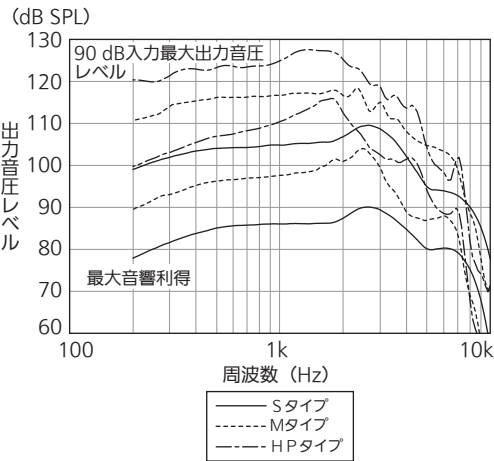
90 dB 入力最大出力音圧レベル周波数レスポンスと 最大音響利得周波数レスポンス
