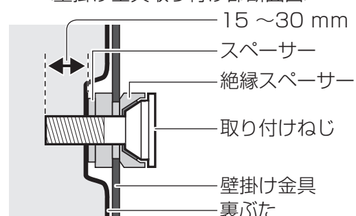
<壁掛け金具取り付け部断面図>
