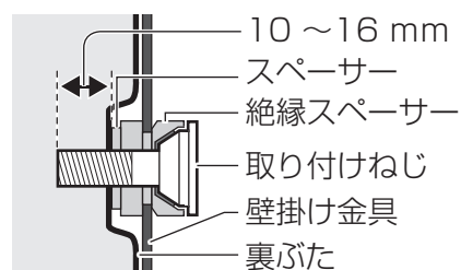
<壁掛け金具取り付け部断面図>
