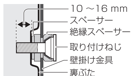
<壁掛け金具取り付け部断面図>
