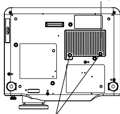
ランプユニット収納扉固定ねじ
