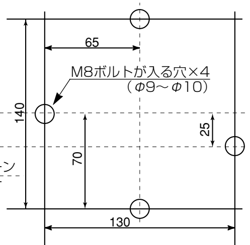
〈取り付け穴寸法〉
