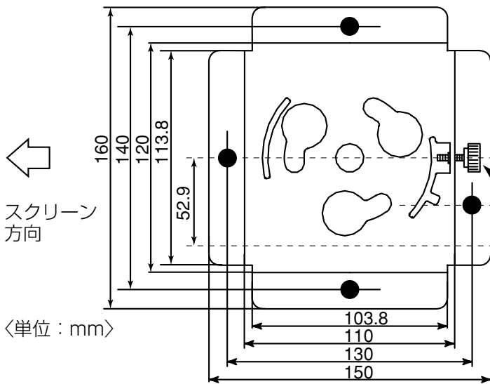
〈アタッチプレート図〉
