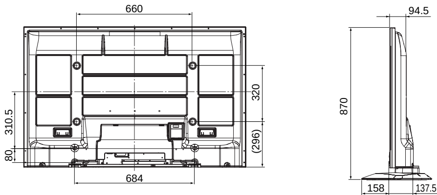
据え置き設置用スタンド取付時
