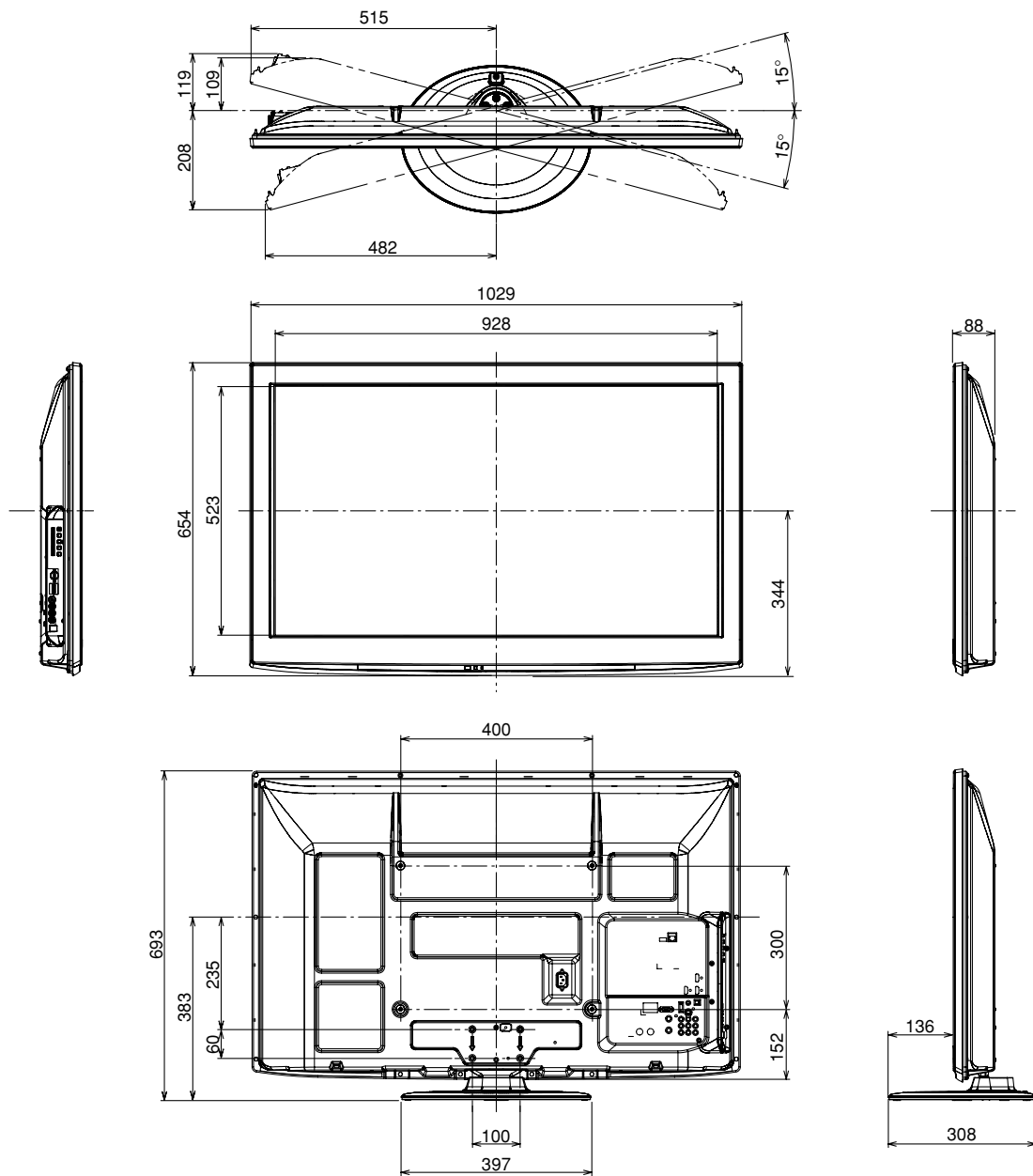
据え置き設置用スタンド取付時
