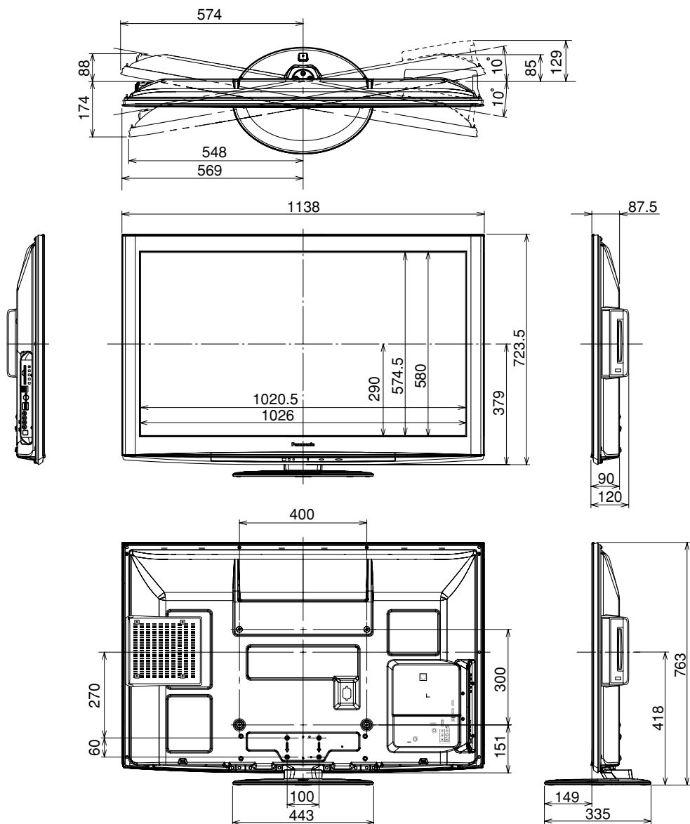
据え置き設置用スタンド取付時
