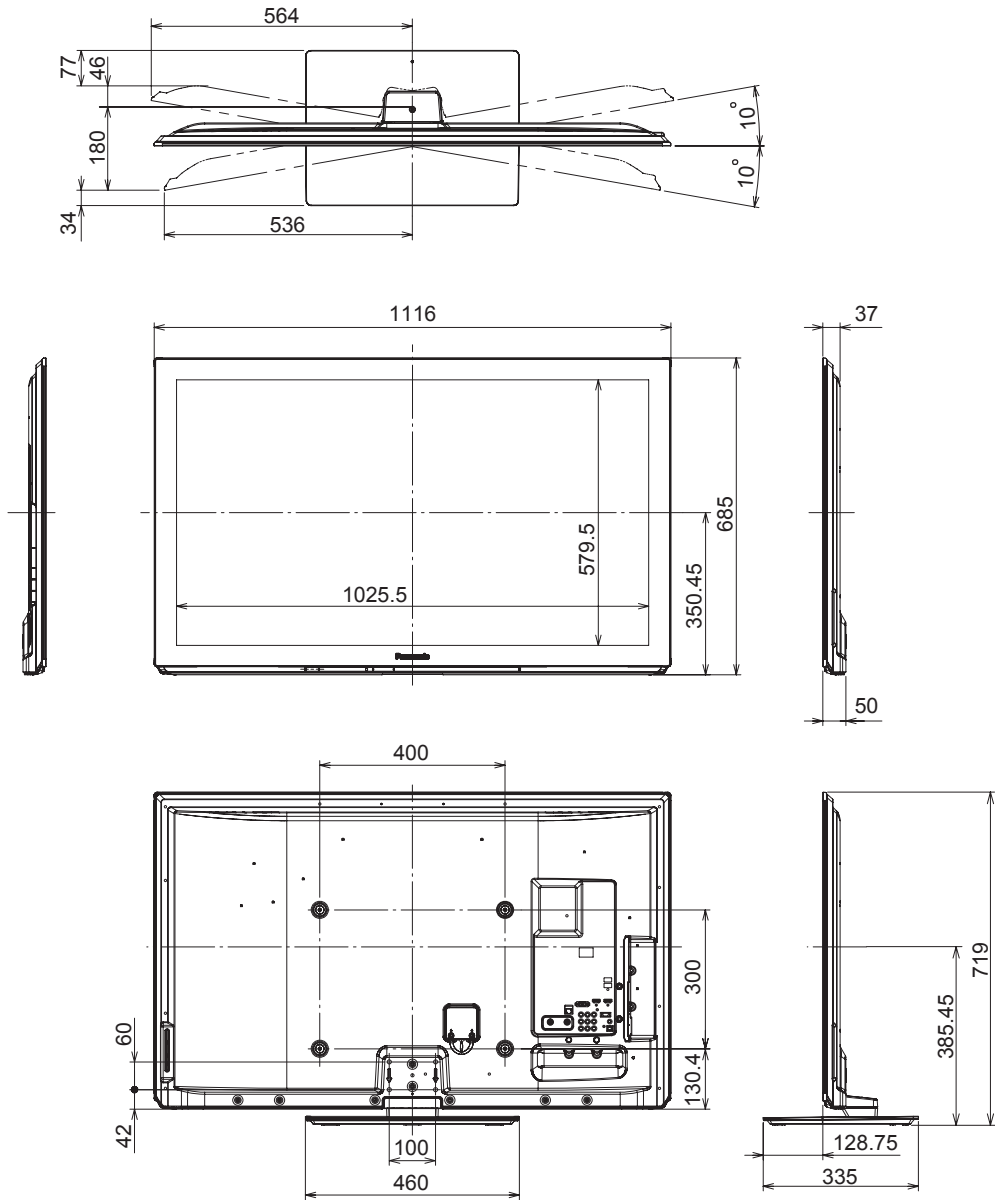
据置き設置用スタンド取付時
