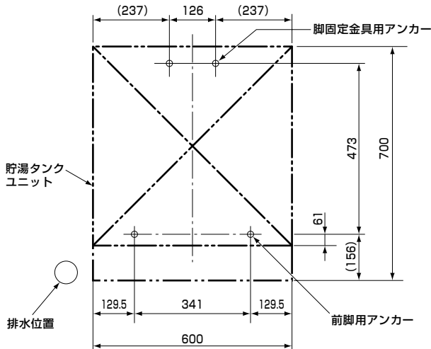
アンカー4箇所とめ
