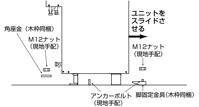
(2) 側面に壁がある場合
