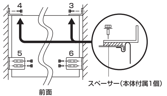
(2) 側面に壁がある場合
