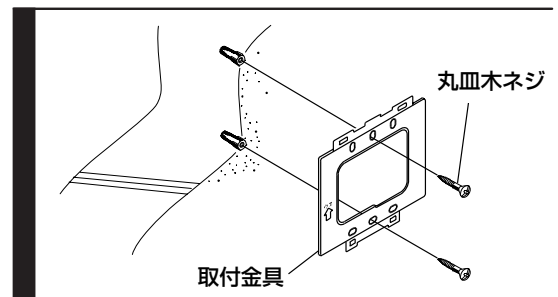
▶▶ 図3 コンクリート壁面への固定の場合
