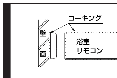
▶▶ 図6 リモコンの周囲をコーキングする
