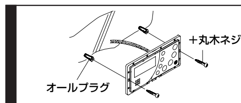
▶▶ 図3 リモコン本体の壁面への固定のしかた
