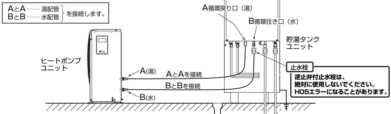
貯湯タンクユニット～ヒートポンプユニット間の配管接続
