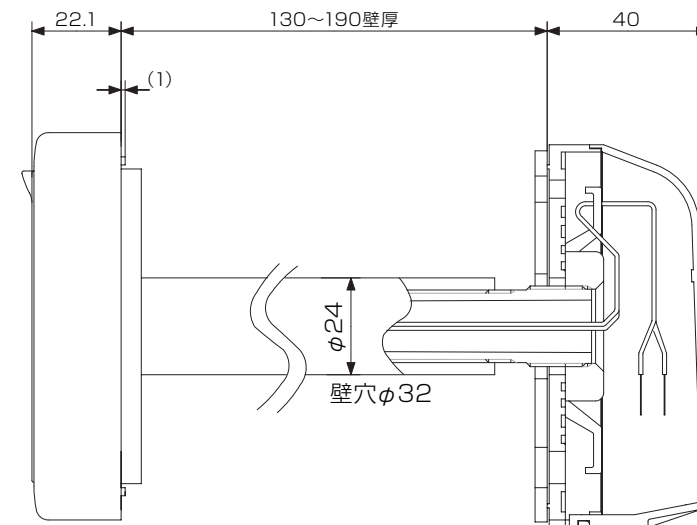
別売品：STK-HPF24CB（風呂リモコン用屋外カバーセット）取付時寸法図
