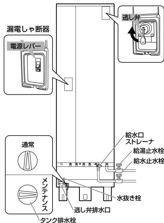
<給水口ストレーナ部>
