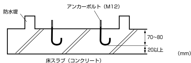
(b)埋込みアンカー工事の場合 工事の施工例を下図に示す
