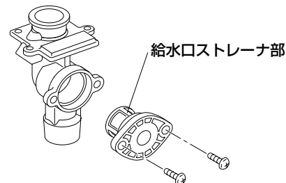
<給水口ストレーナ部>
