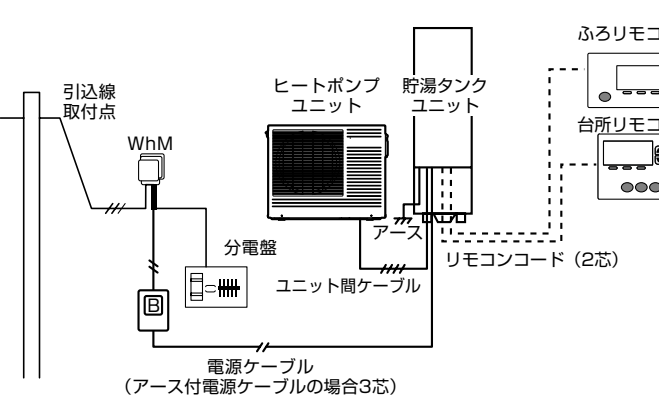
電力量計負荷から配線する方法
