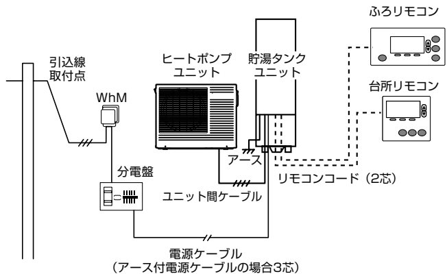
住宅用分電盤から配線する方法
