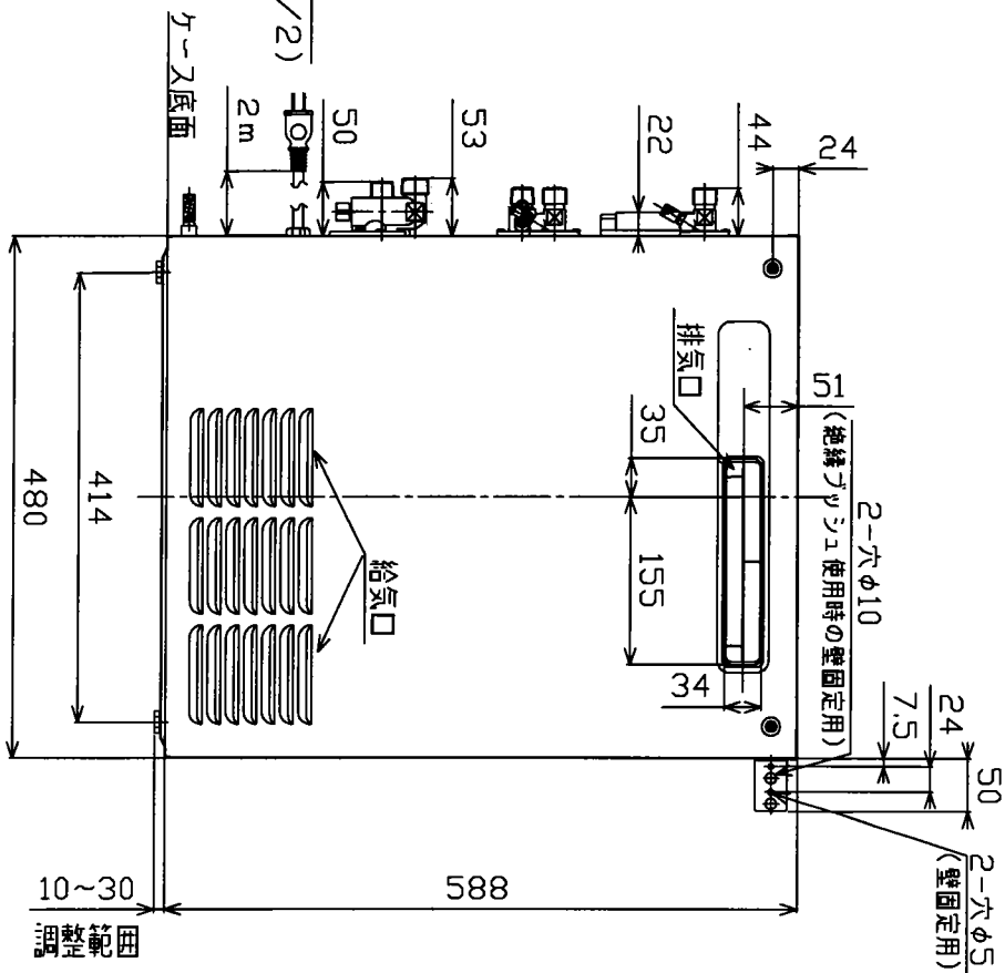
＜正面図＞
