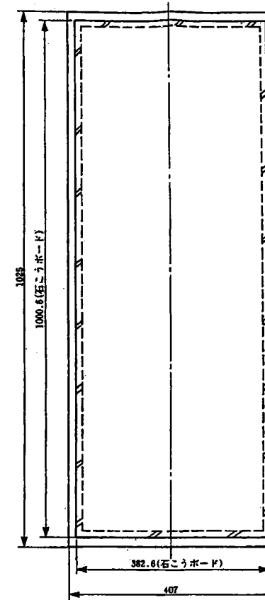
《裏面図》
