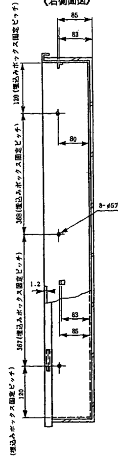
《右側面図》
