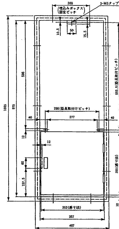
《正面図》
