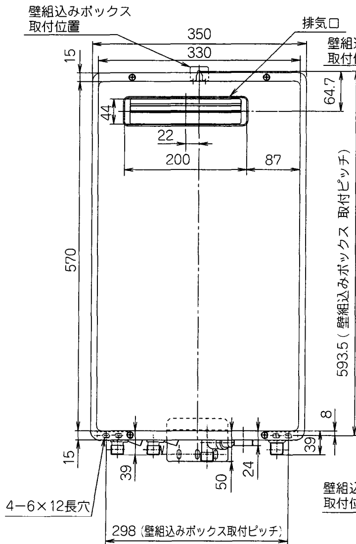
〈正面図〉
