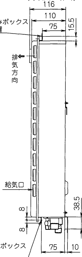
〈右側面図〉
