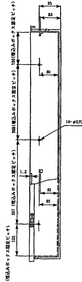
〈右側面図〉
