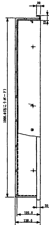
《左側面図》
