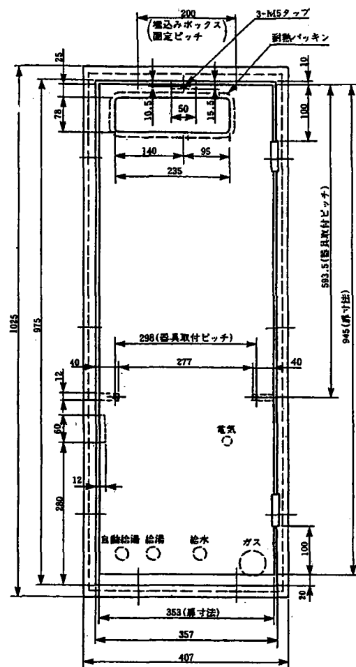
《正面圖》
