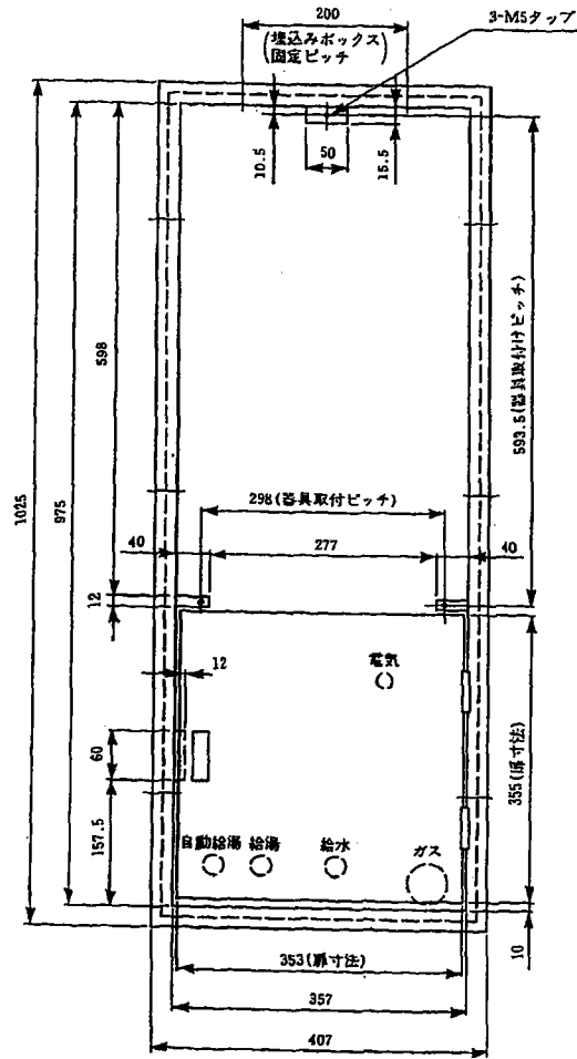
〈正面図〉
