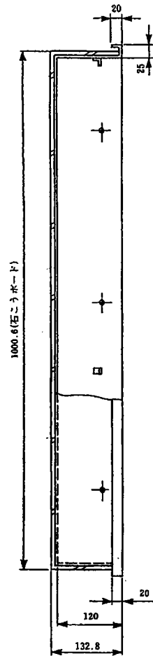
《左側面図》
