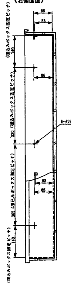
《右側面図》
