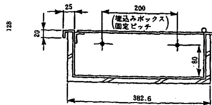
〈下面図〉
