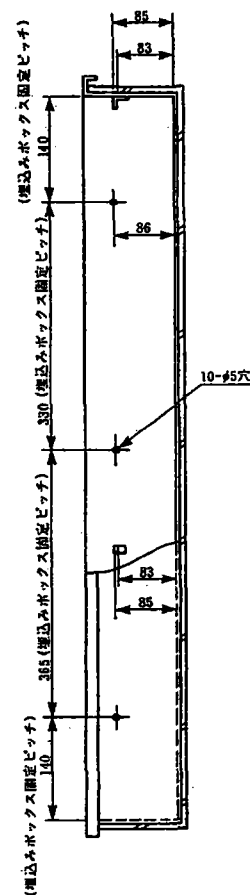
《右側面図》
